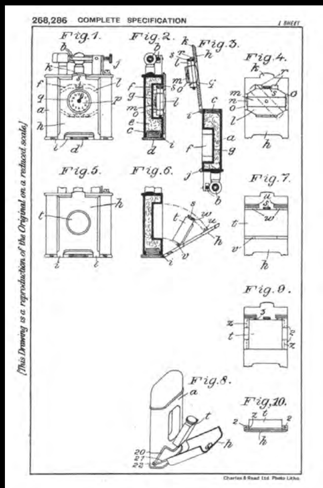
Рисунок из британского патента №268286
